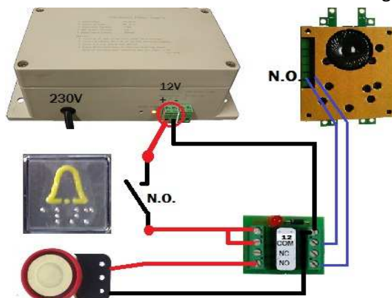
ALARMPIEZO MET N.O. DRUKKNOP IN DE LIFT
