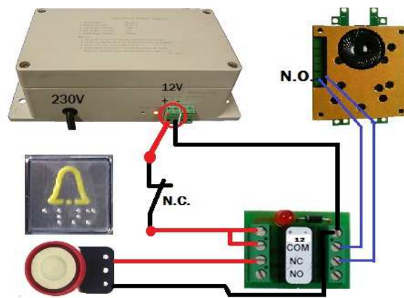
ALARMPIEZO MET N.C. DRUKKNOP IN DE LIFT
